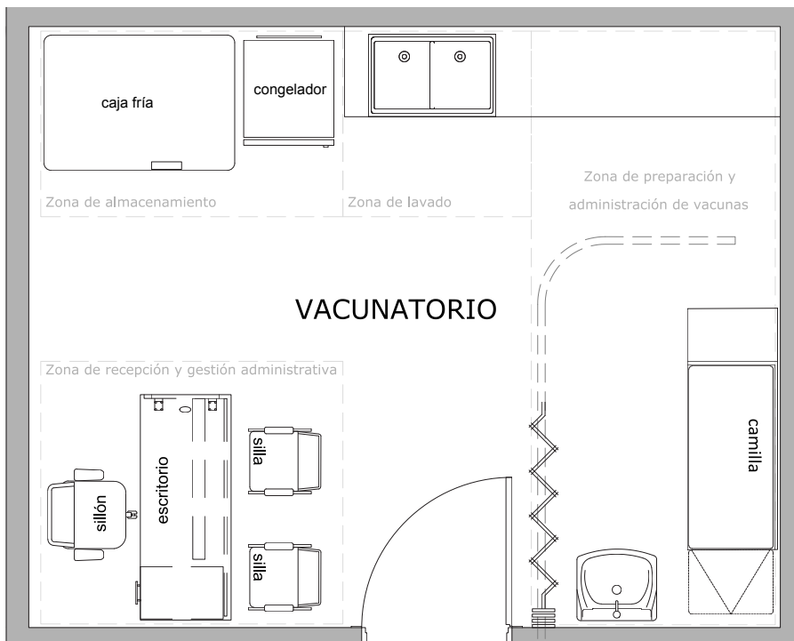
Ilustración 4. Organización del vacunatorio y zonas mínimas requeridas.
