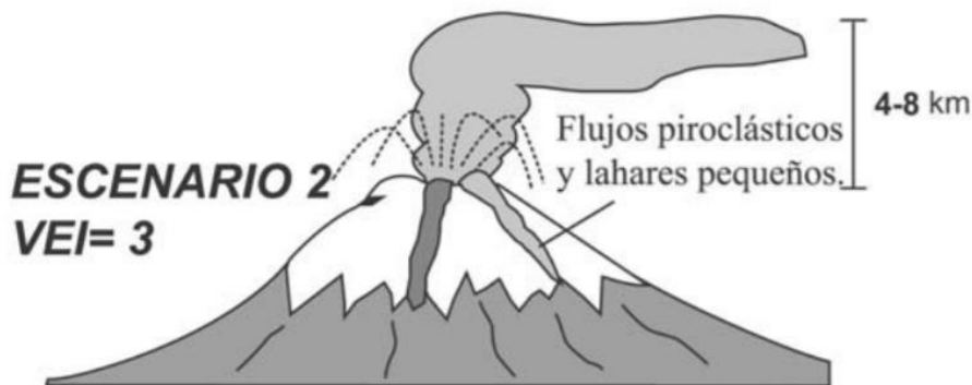
Figura 3 Escenario 2 Lahares pequeños y flujos piroclásticos producto del proceso eruptivo del volcán Cotopaxi
